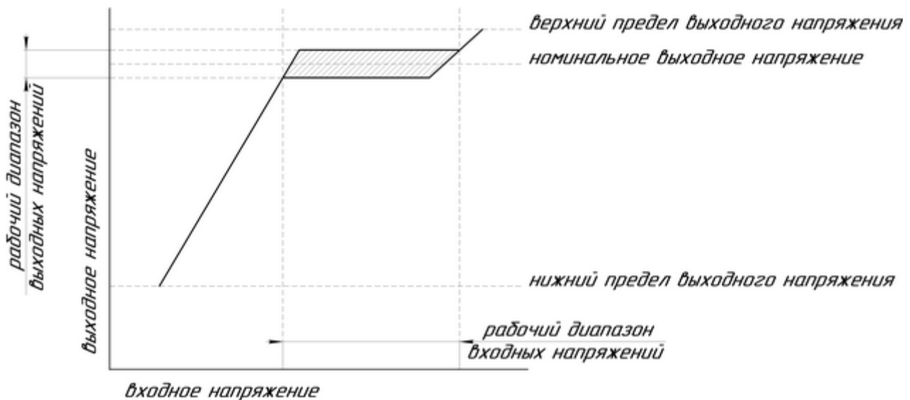
Рисунок 1. Передаточная характеристика стабилизатора напряжения.
